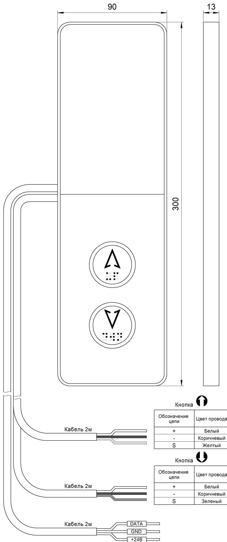
Рис.1 Внешний вид Вызывной пост ОНИКС НШЕК.468381.028
